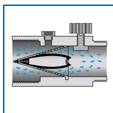
Il setaccio a cono Inox protegge la vostra attrezzatura.
