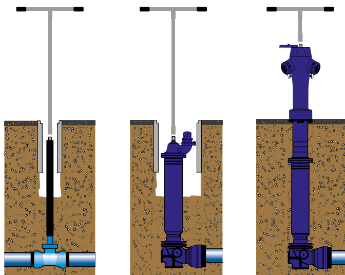
Chiave di fontaniere VARIO per applicazioni diversi.
